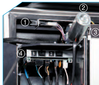
1) Safety microswitch 2) Motor 3) Encoder 4) Lift card
